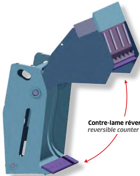
Avec contre-lame avant With front counter plate G4X1.A
